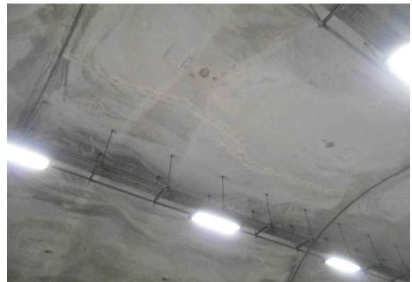
라이닝 SPAN.57 균열(0.3mm 미만)
