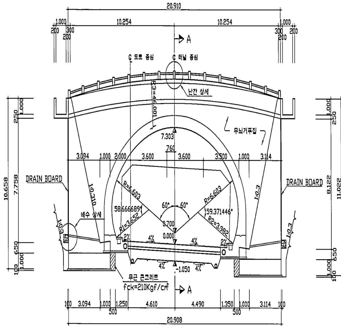
정 면 도 (춘천방향)
