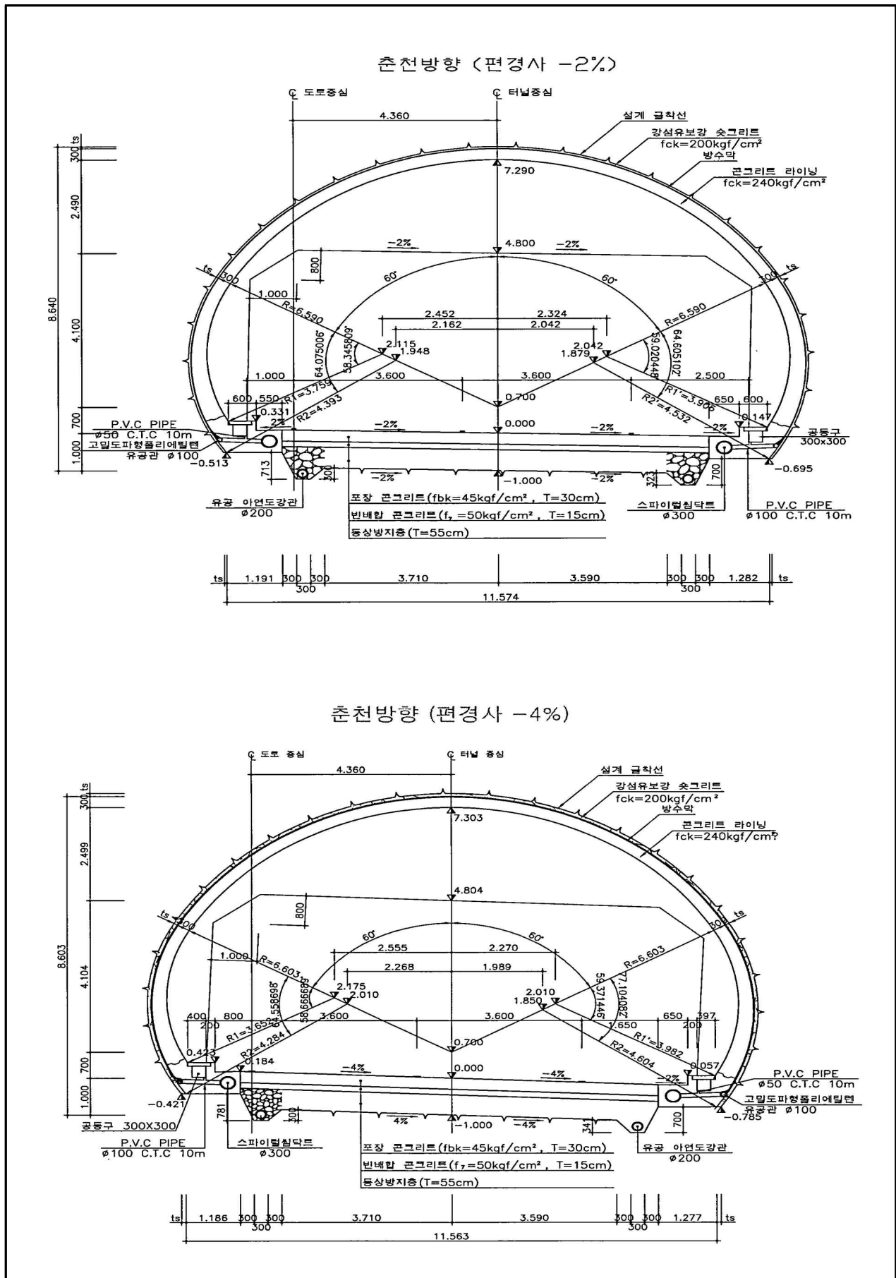
<그림 2.1.5> 횡단면도(표준단면도-동상방지층)
