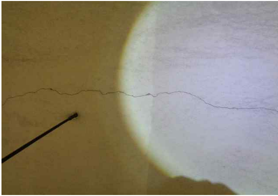
라이닝 SPAN.36 균열(0.3mm 이상)
