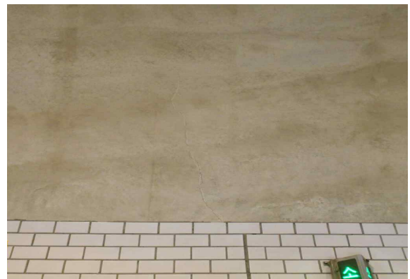
라이닝 SPAN.66 균열(0.3mm 미만)
