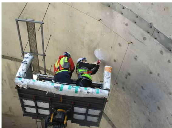
반발경도 측정 현황(천단부)
