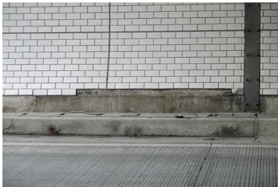
측벽부 SPAN.1 타일탈락
